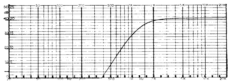
D Réponse de la sortie aiguë.
