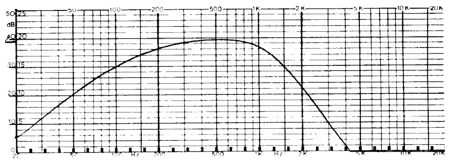
C Réponse de la sortie grave avec coupure des fréquences inférieures à 150 Hz.
